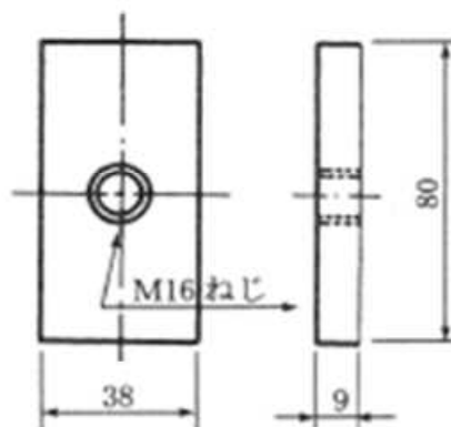
① インサートナット
