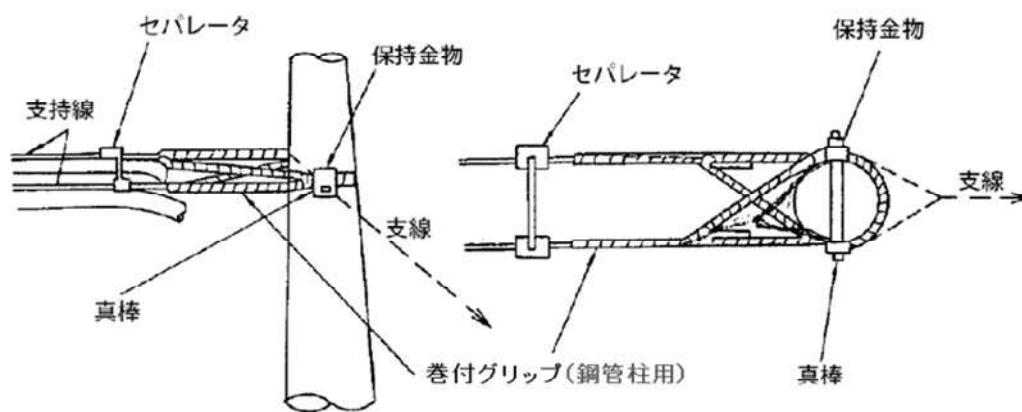
平行引留め
