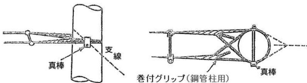
平行引留め
