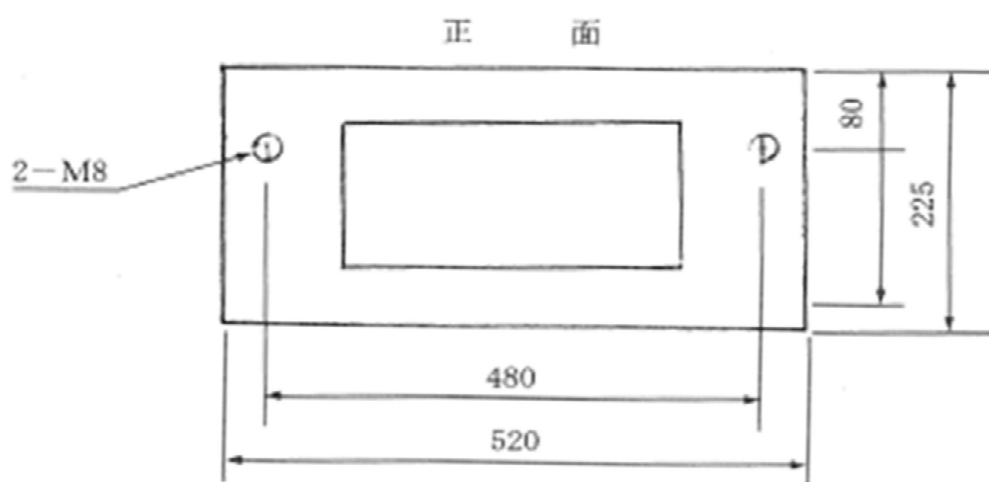
機器上面図
