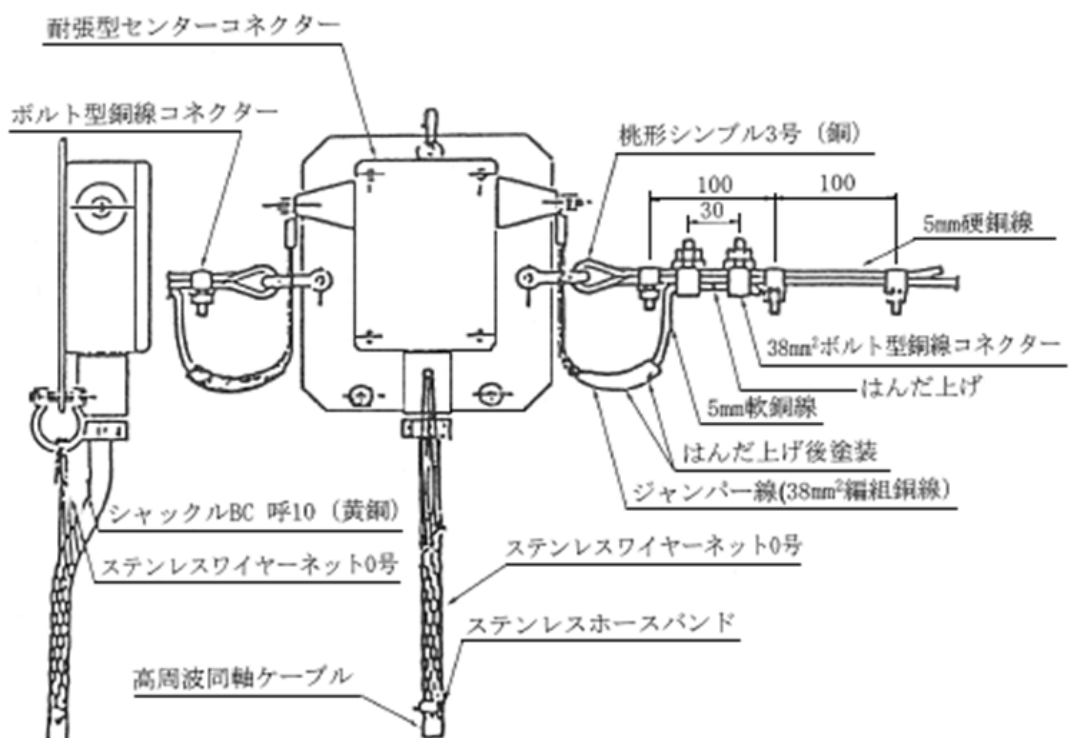
参考資料 3 図 1.2.6-4 E 部詳細 (整合トランス付直張り)
