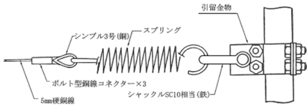
参考資料 3 図 1.2.3 A'部詳細図 (スプリング挿入の場合)
