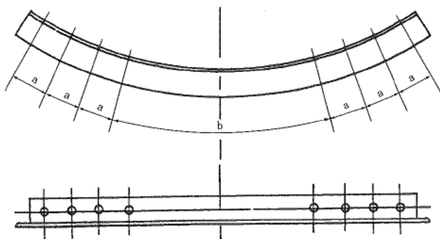
アンテナ架台取付部材（下部）
