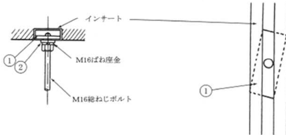
① インサートナット
