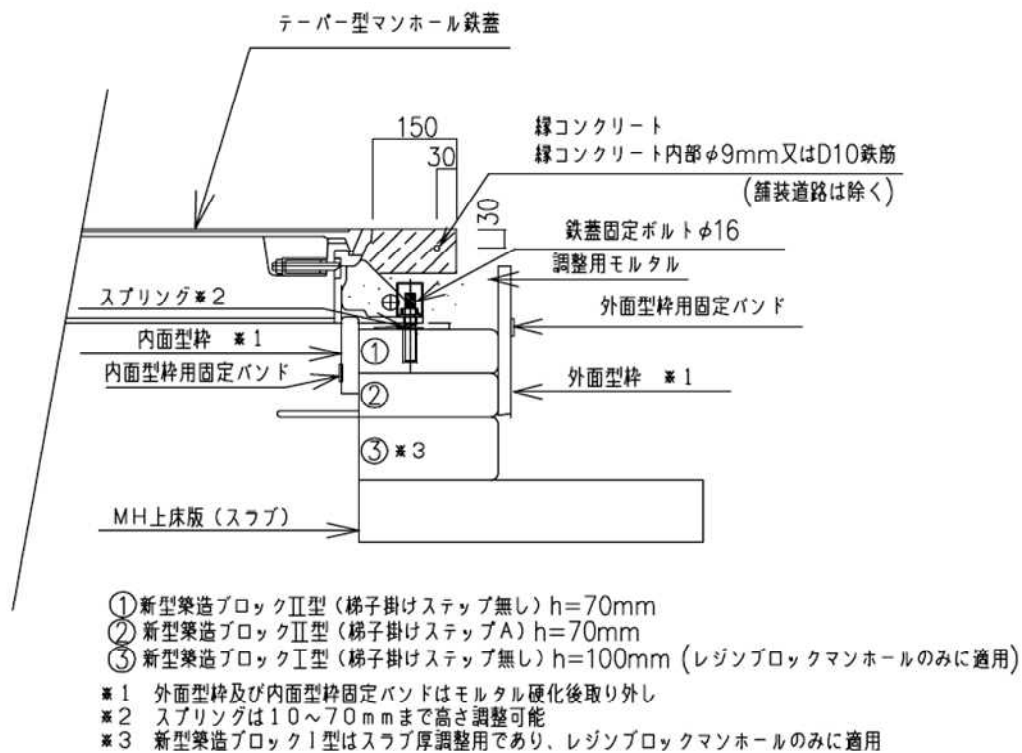
首部構造 (単位: mm)
