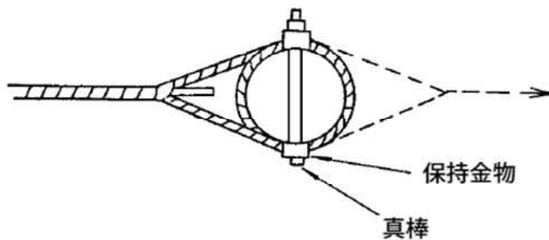
1 条引留め
