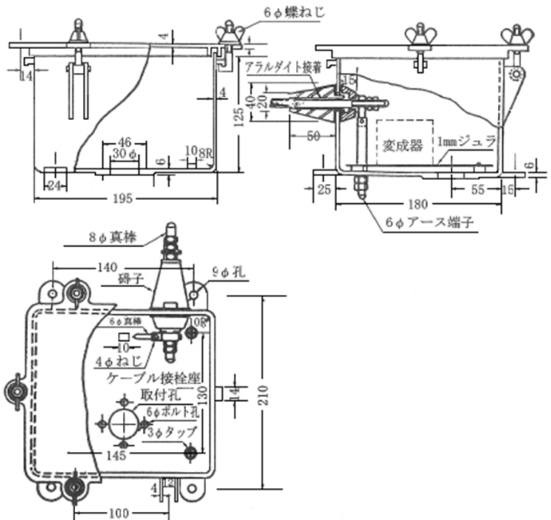
参考資料 3 図 1.3.1 空中線整合箱（傾斜型、逆L型、ホイップ型用）
