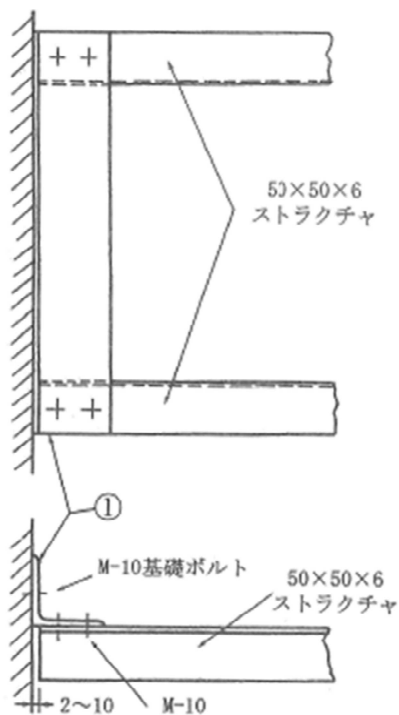
①ストラクチャ取付金物
