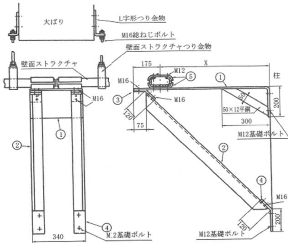
柱面から離して取付ける場合 (251~700mm) ①
