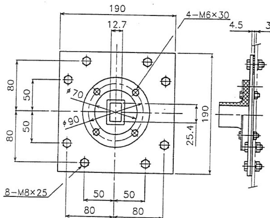
图 6-3 WR J-10 方形导波管贯通金物 (1 条横壁用)
