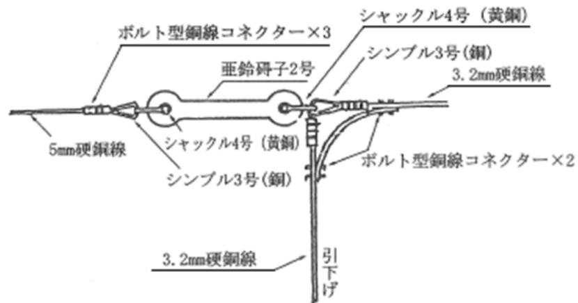
参考資料 3 図 1.2.14 O部詳細
