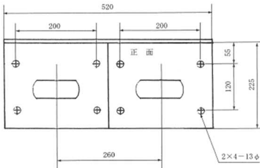
無線機底面
