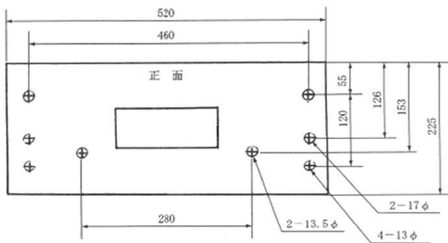
搬端底面
