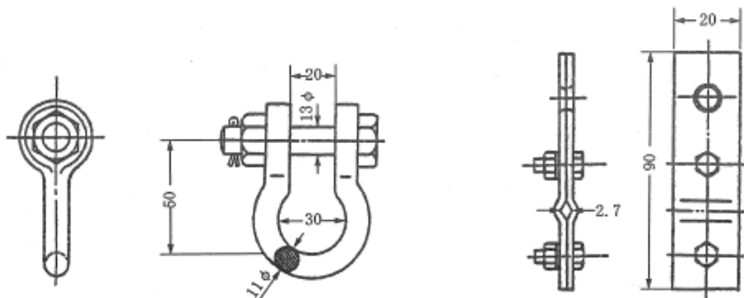
付図 11 桃形シャックル
