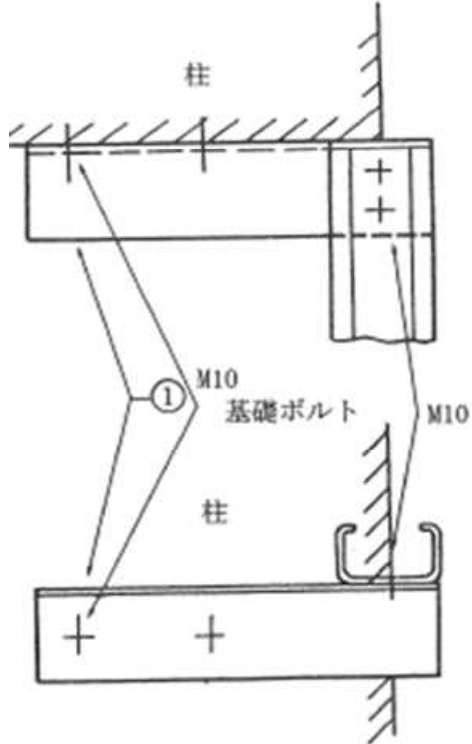
(B) リップ溝形鋼の場合
