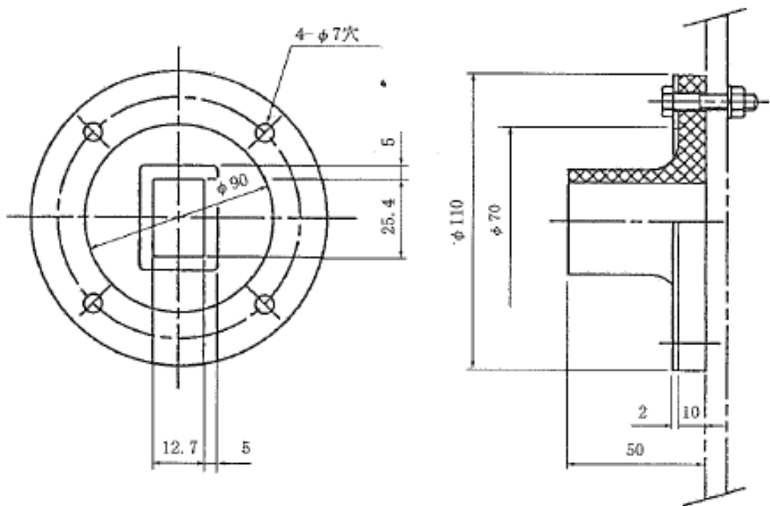
图 6-7 WRJ-7 方形导波管贯通金物 (1 条天井用)
