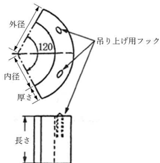
コンクリートブロックの構造
