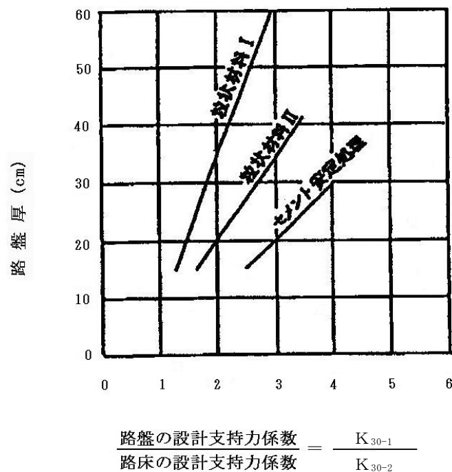
図 4－4 路盤厚の設計曲線
