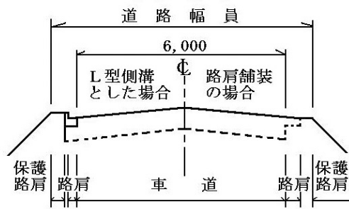
図 2 - 3 B 種道路
