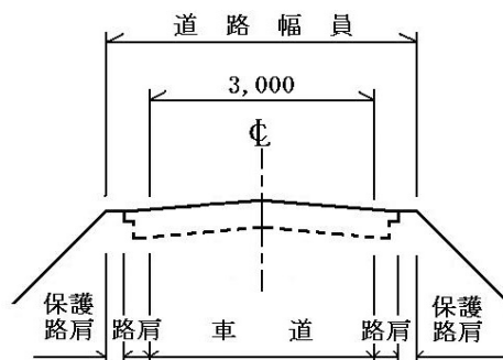
図 2 - 6 E 種 道 路
