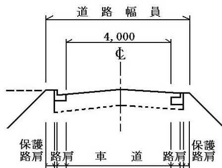
図 2 - 5 D 種 道 路
