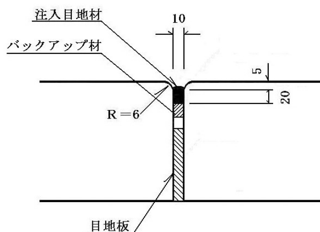
図 4－13 膨 張 目 地
