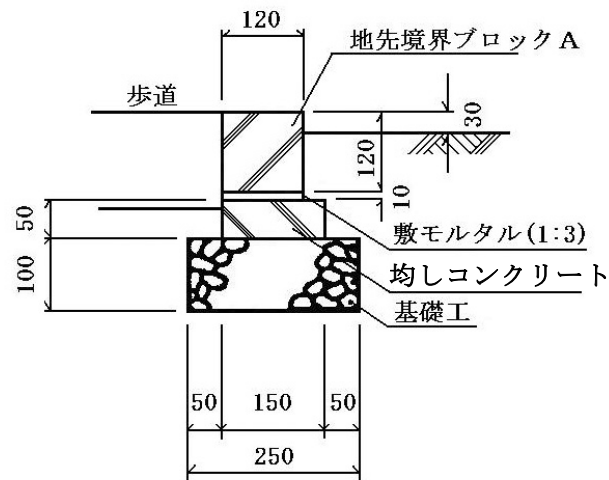
図4-18 舗装止め工
