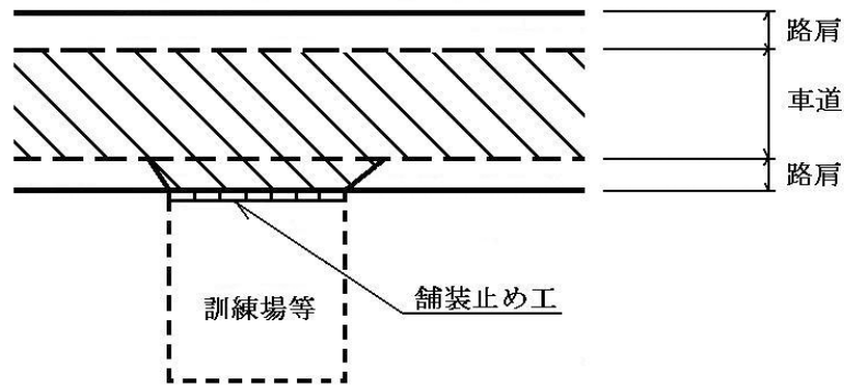
図4-20 舗装止め工設置位置
