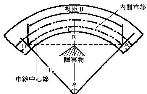
図 2-7 視距の確保
