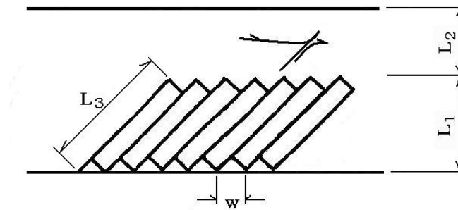
(c) 45° 後退駐車
