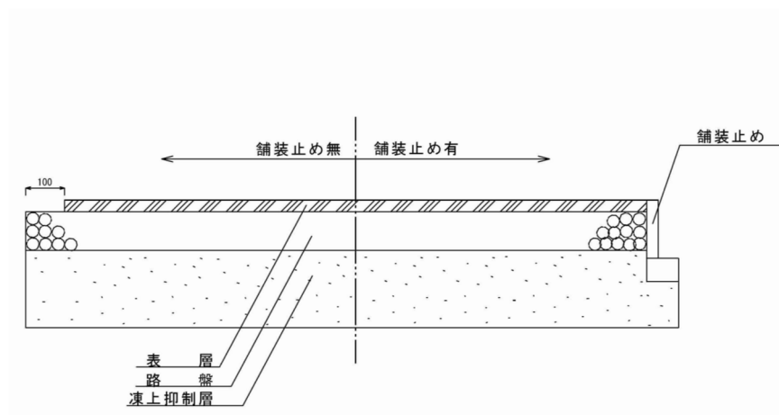
図 4－17 アスファルト歩道の構成と名称
