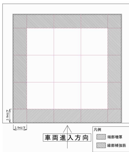
図4-7 設計例
