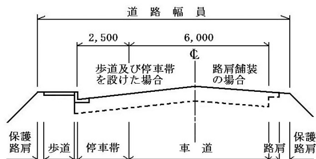
図2-2 A種道路
