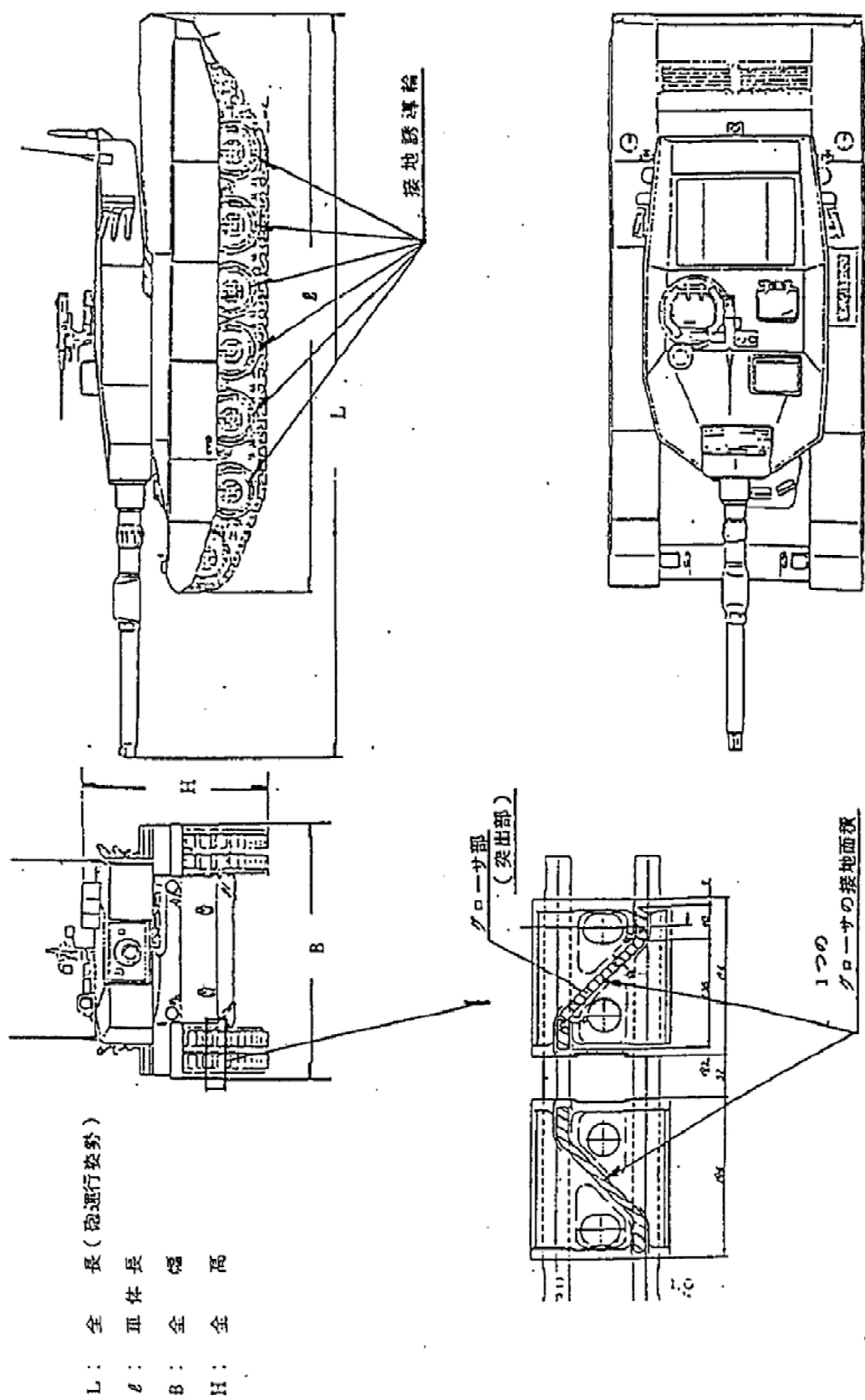
図 7 - 2 車両諸元図
