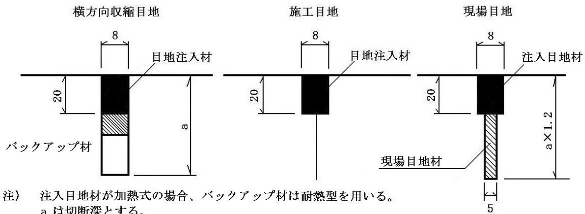
図 4－12 目地の寸法
