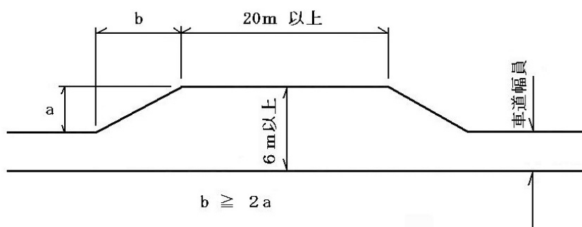
図 2-11 待避所の形状
