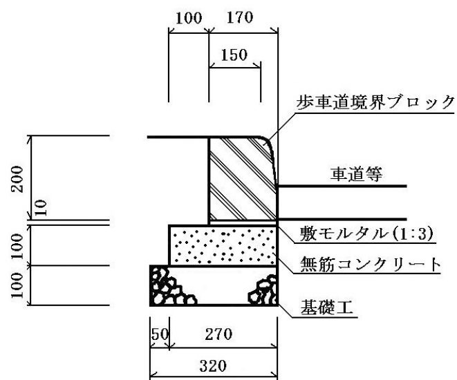
図 4-22 縁 石 工
