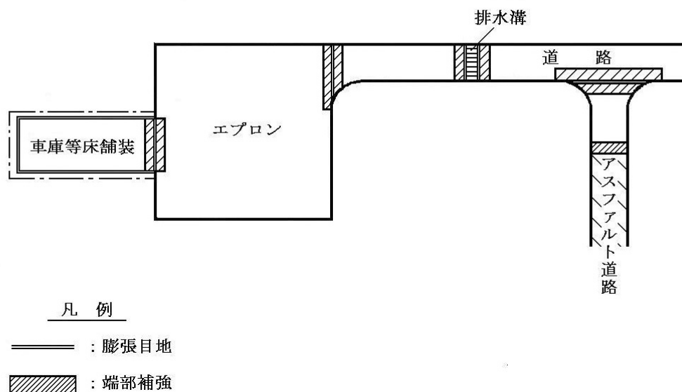
図 8－2 道路舗装の端部補強箇所
