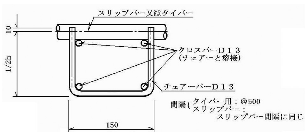
図 4-11 チェアー
