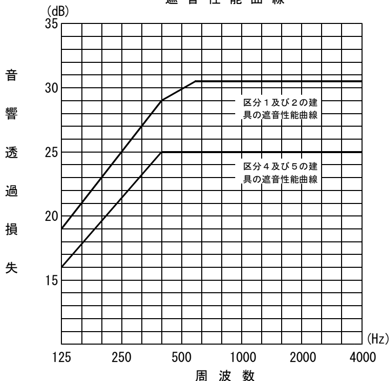
遮音性能曲線
