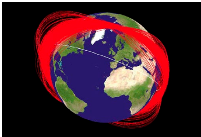
中国衛星迎撃実験により生じたデブリ（一か月経過） ※白線は国際宇宙ステーションの軌道【NASA】
